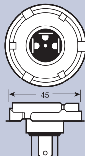
P45t IEC 7004-95 DIN 49737
